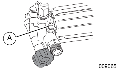
Figure 2-7. Fixation du tube de siphonnage
