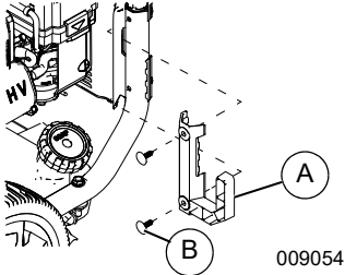
Imagen 2-3. Instalación del gancho de la lanza
