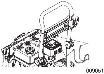
Figure 2-4. Installation du crochet du tuyau
