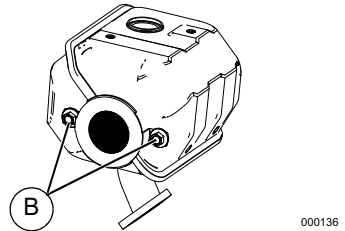
Figure 4-10. Attaches du pare-étincelles
