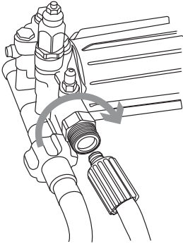
Imagen 2-13. Conexión de la manguera de alta presión a la bomba
