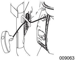
Imagen 2-6. Instalación de la cuerda de retroceso
