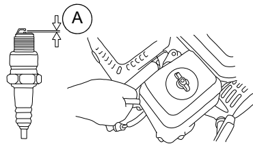
Imagen 4-8. Bujía
