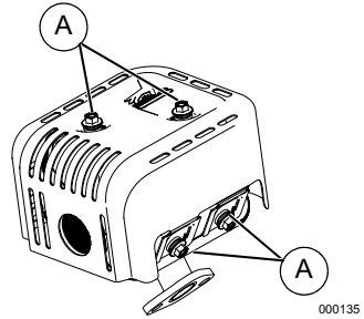
Imagen 4-9. Fijaciones del protector de calor
