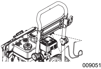
Imagen 2-4. Instalación del gancho de la manguera
