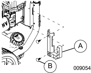
Figure 2-3. Installation du crochet de lance
