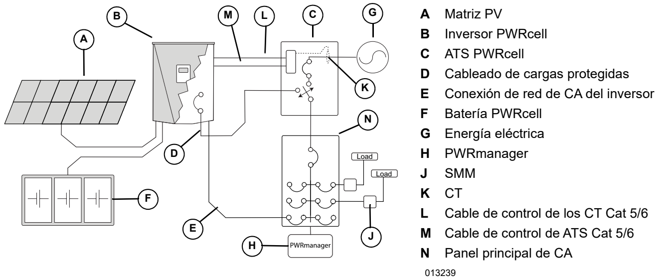
Figura 5-9. Reserva para todo el hogar
