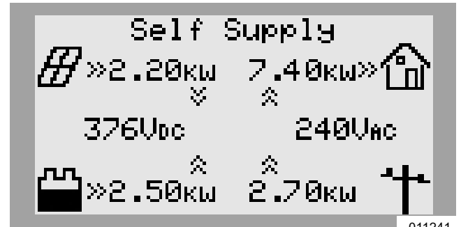
Figura 7-24. Self Supply (Autoabastecimiento) (3 de 3)
