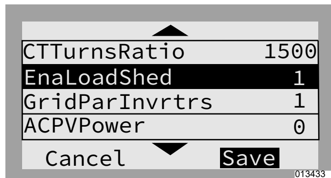
Figura 7-21. PV + Almacenamiento: Todo el hogar (3 de 3)
