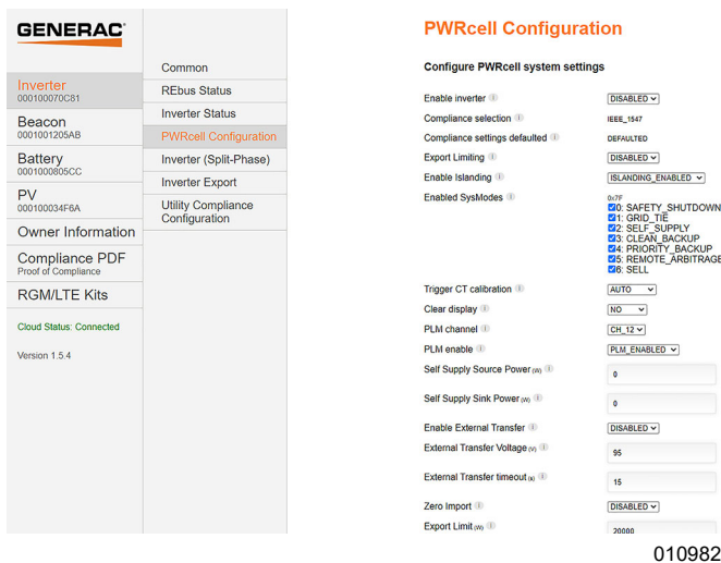
Figura 6-29. Configuración de PWRcell
