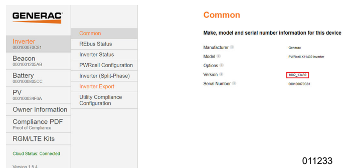
Figura 6-30. Verificación del firmware del inversor
