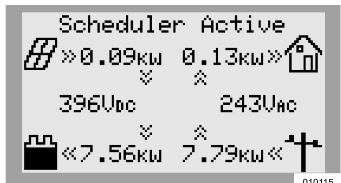
Figura 6-20. Programador activo
