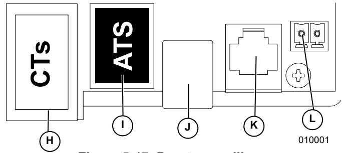
Figura 5-17. Puertos auxiliares
